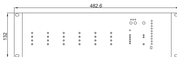
Fig1. Dimensioni per il montaggio
