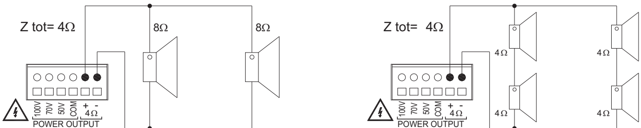
Fig7. Linee a Impedenza Costante
