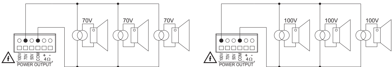
Fig6. Linee a Tensione Costante
